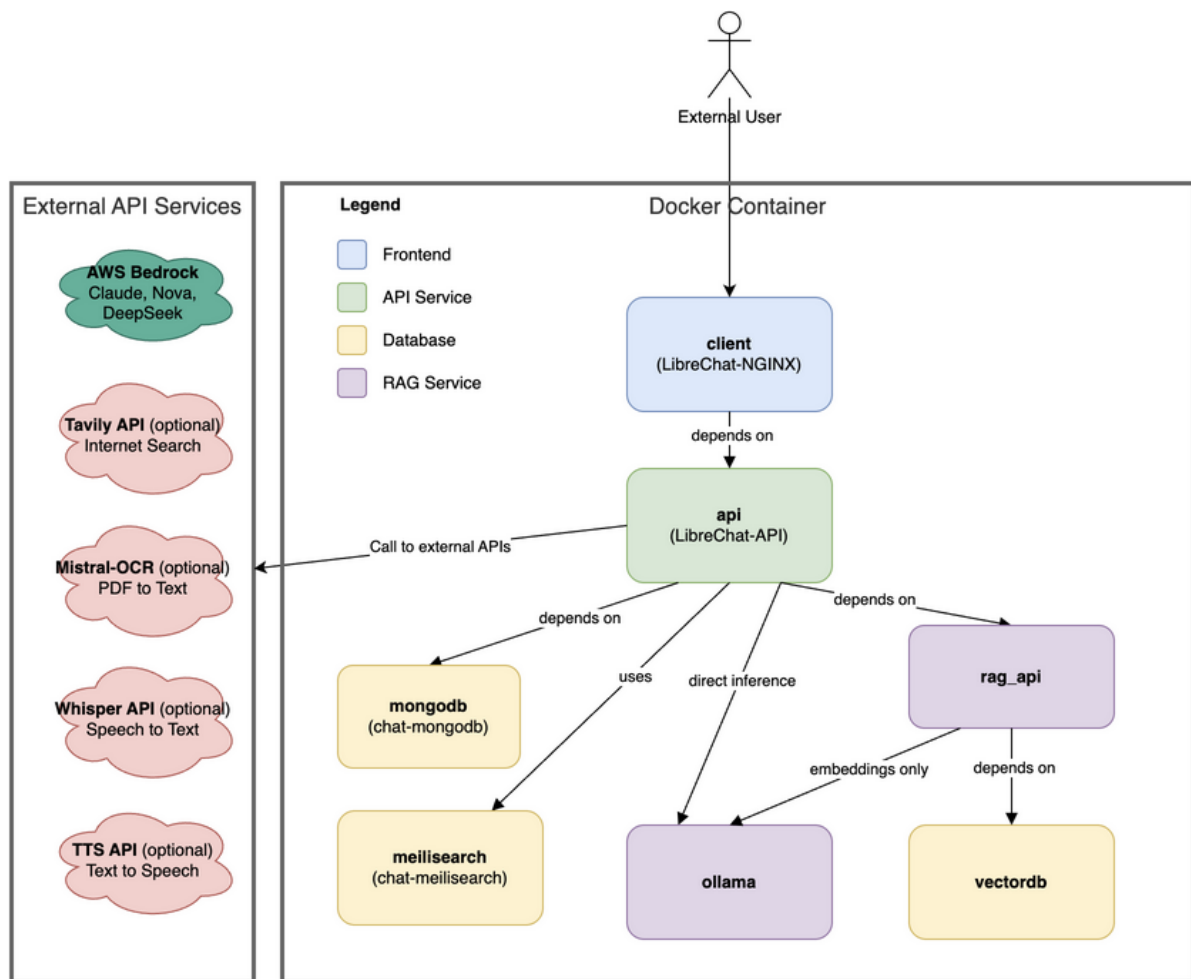
Figure 2: Kernarchitektur, die allen Private AI-Bereitstellungen zugrunde liegt und konsistente Leistung und Skalierbarkeit gewährleistet.
