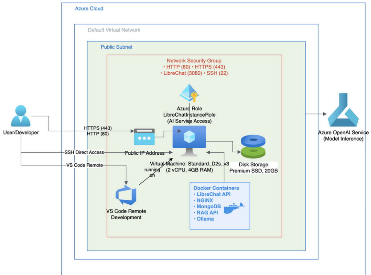
Figure 4: Azure-Architektur mit OpenAI-Modell-Integration, die kohäsive Kompatibilität mit Microsoft-Services für Private AI bietet.
