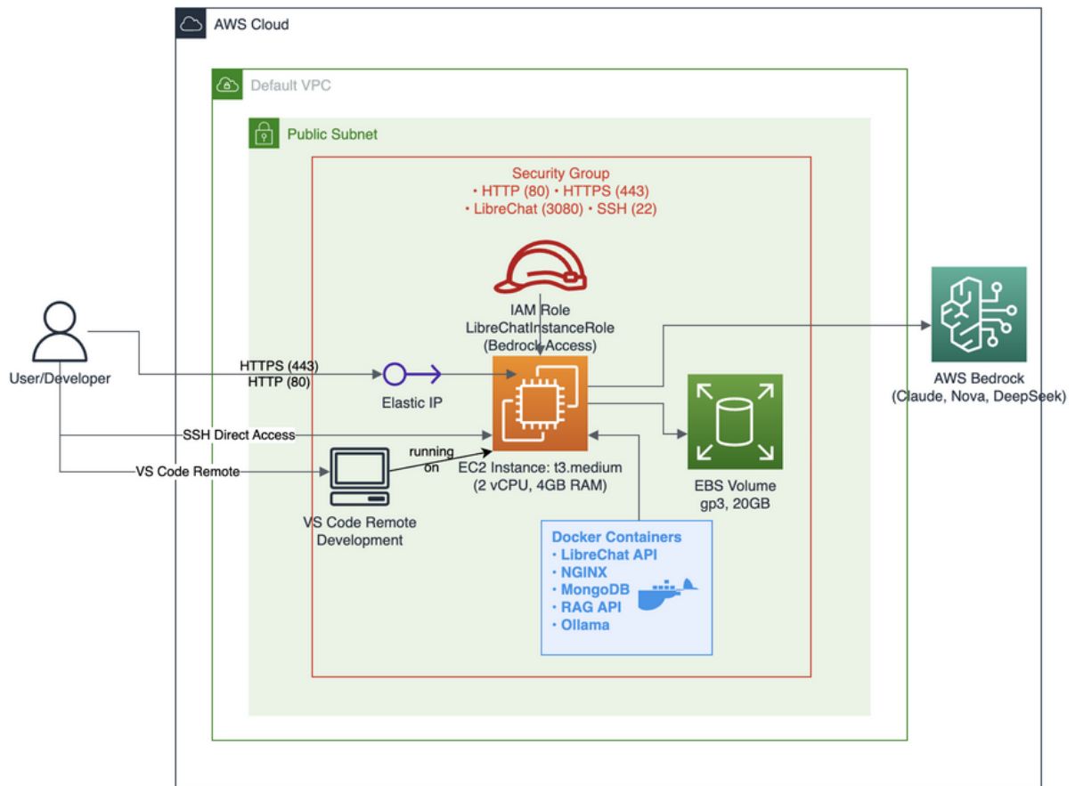
Figure 3: AWS-Architektur mit Bedrock-Integration, entwickelt für nahtlose und schnelle Private AI-Bereitstellung.
